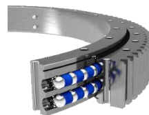
ДВУХРЯДНЫЕ ОПОРНО- ПОВОРОТНЫЕ ШАРИКОПОДШИПНИКИ (Тип K2)
