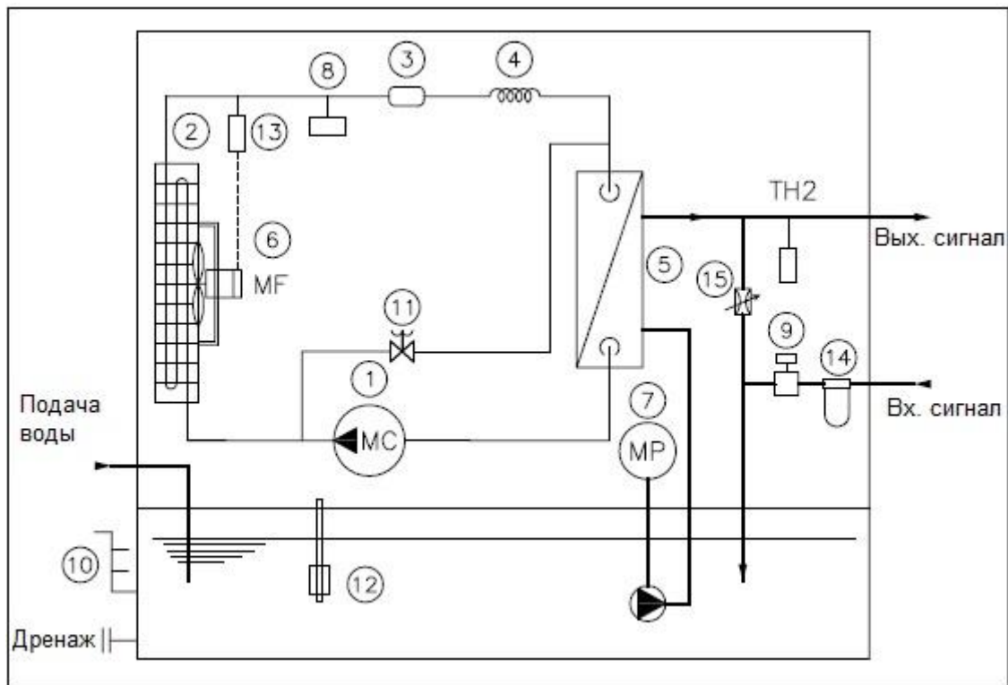
Иллюстрация 12: Гидравлическая система охладительного узла (HWK-V серии)
