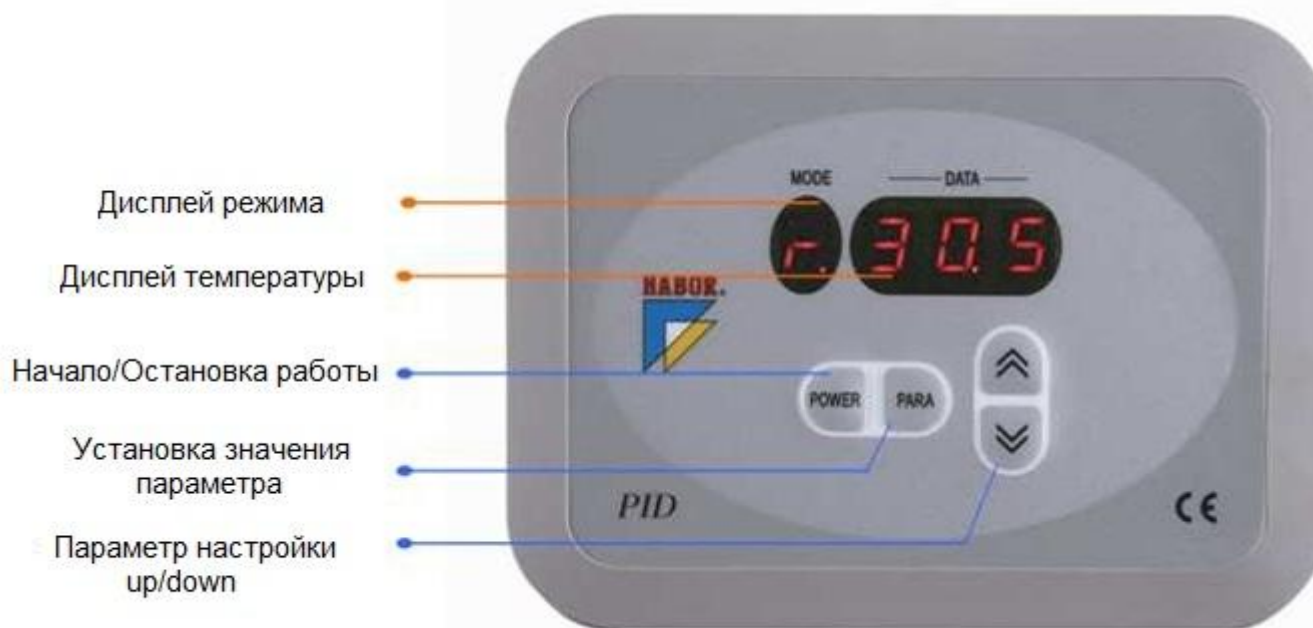
Иллюстрация 8: Дисплей панели ПИД-управления
