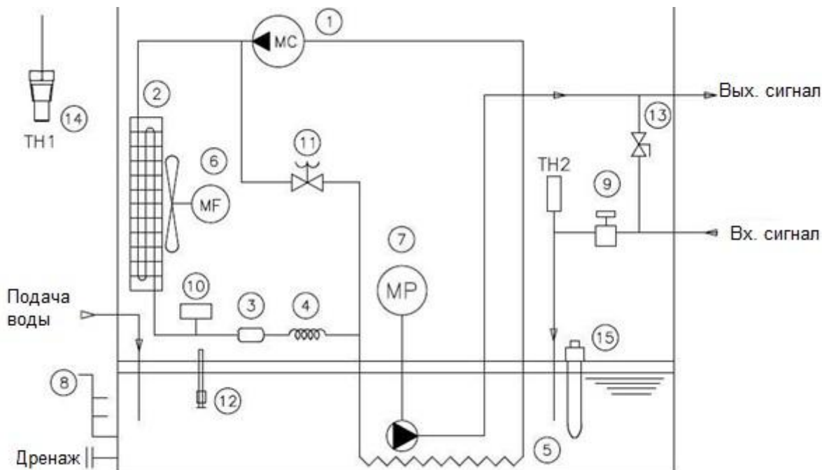
Иллюстрация 13: Гидравлическая схема для охладителей, оборудованных стандартным температурным управлением (оснащенных баком)
